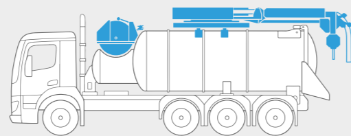
HELICOPTER 360-60T TANDEM pour aspiration et curage
